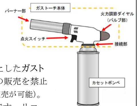
ガストーチの構造例
