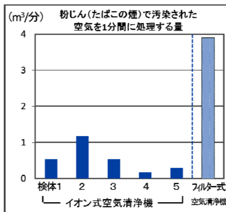
図10 集じん能力の比較
