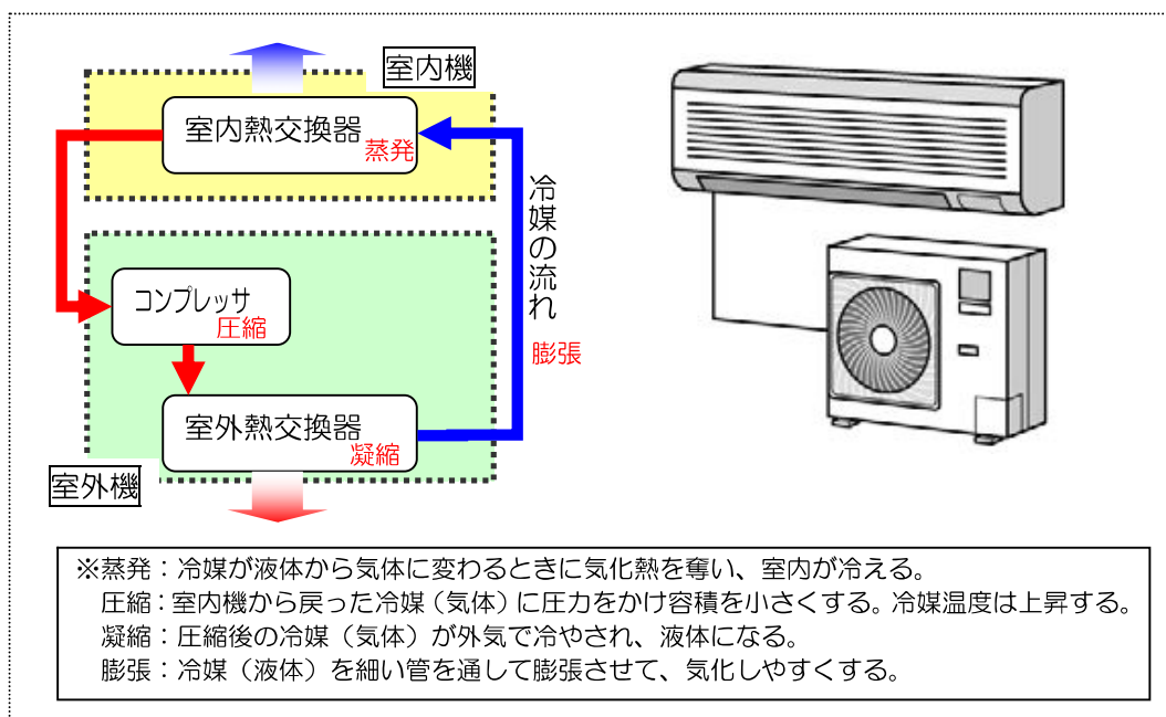
図2-2 エアコンの冷却の仕組み
