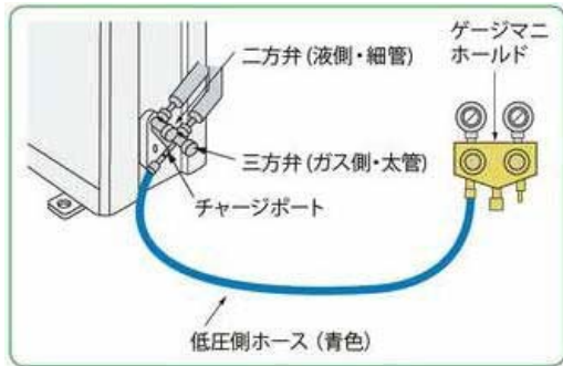
図2-4 ゲージマニホールド： 冷媒の気化状況のチェックやガス充填作業等に使用する圧力計の一種。
