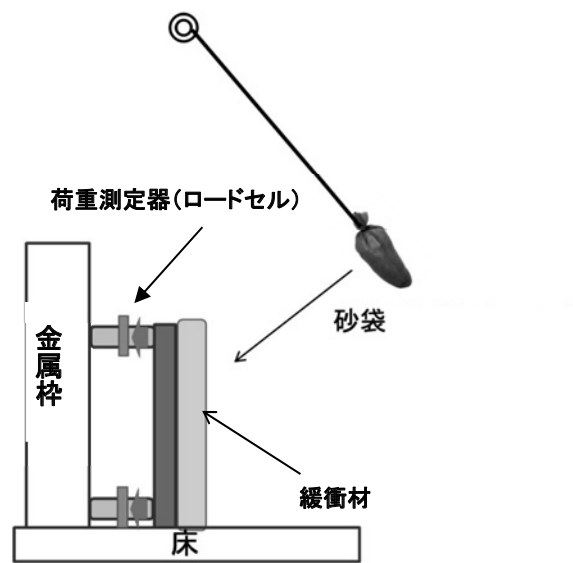
図 7-3 砂袋を使った衝撃力測定試験のイメージ図（緩衝材有）
